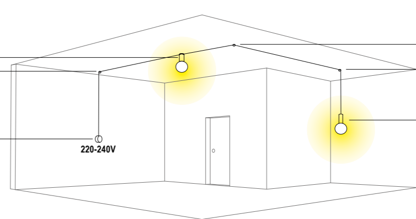
0605 Deviatore e decentratore Displacement element
