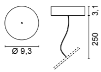
0946 Rosone completo di cavo di alimentazione. Ceiling rose with cable. .01 Bianco - White
