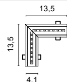
0957 Angolo 90° - 90° corner
