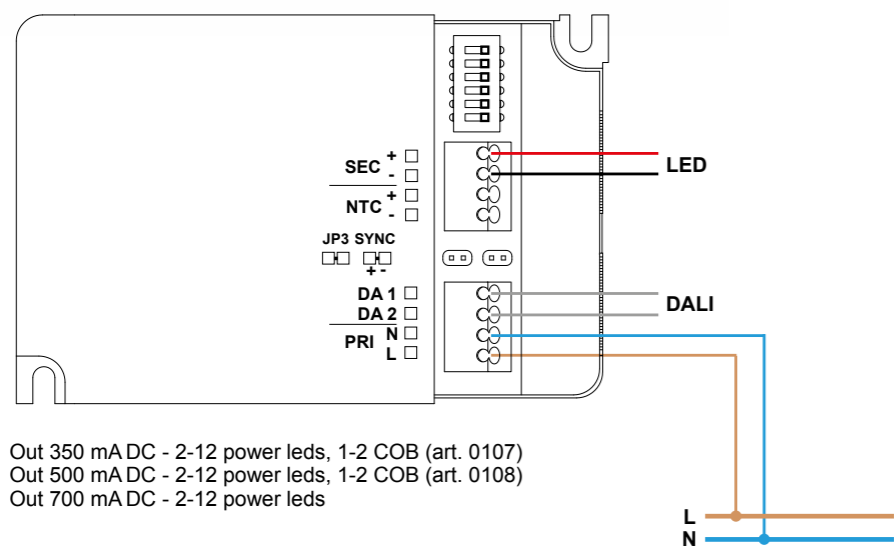
0129/DALI
