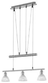
Pendelleuchte · Pendant ↔ 60,5 cm, ↓ 95 - 160 cm incl. 3 x LED E14, 5 W 3 x 400 lm, 3.000 K
