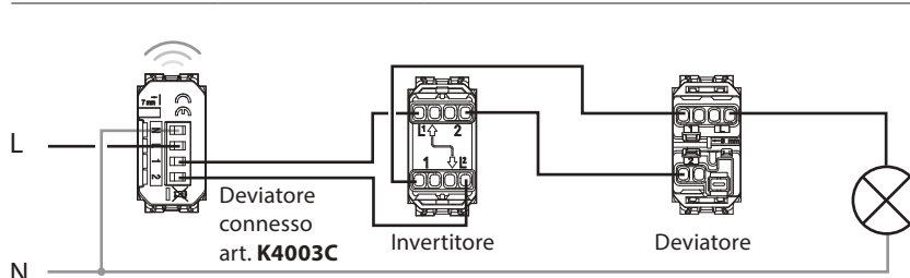
Schema di collegamento - deviato o invertita
